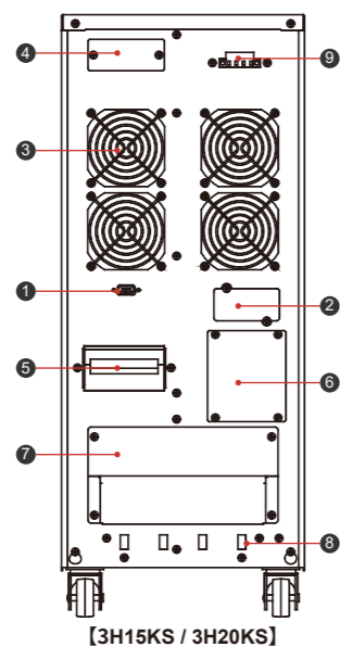
[3H15KS / 3H20KS]
