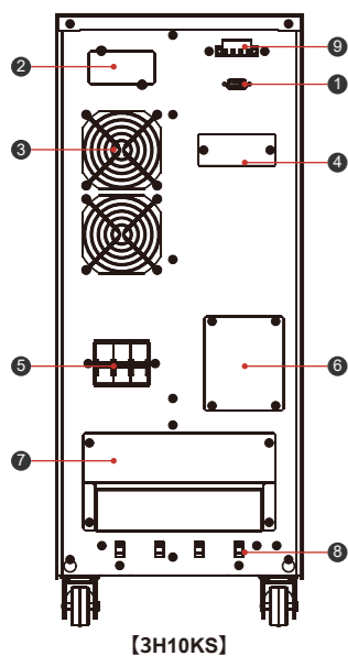
[3H10KS]
